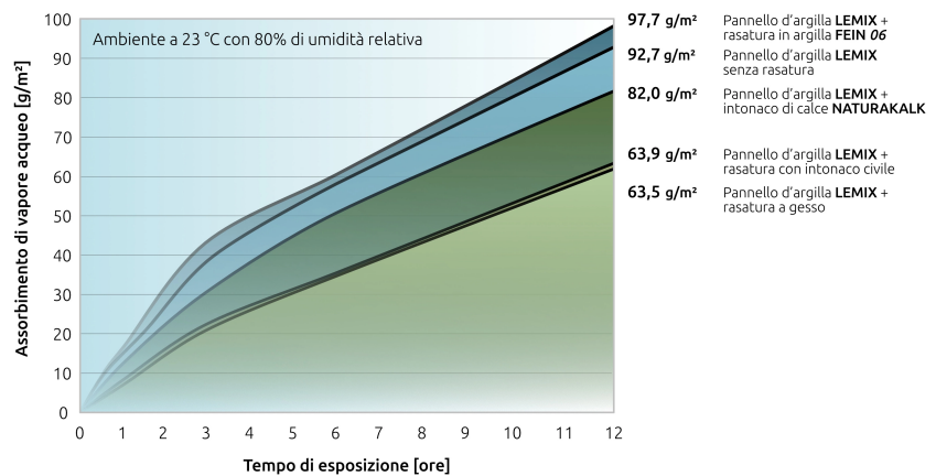
Assorbimento dell'umidità dell'aria - pannello Lemix con finiture diverse
