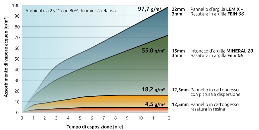
Assorbimento dell'umidità dell'aria per tipologia di rivestimento interno
